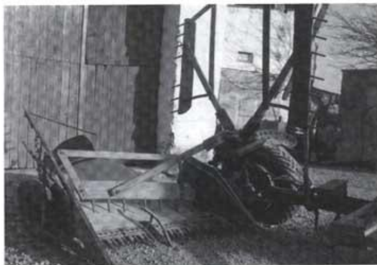
Màquina de segar. Anava enganxada al matxo o mula i els mecanismes de segar i els de amuntegar la palla s'accionaven al voltar la roda. Aquesta és de la marca "Trepit" fabricada en Tàrrrega (Lleida). N'hi ha unes altres de la marca "Ajuria" fabricades a Vitòria.
