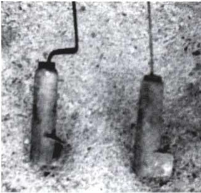
Corbella i falç. Es pot apreciar la diferència del mànec de les dues peces. La fulla de la falç ix en el mateix pla que el mànec. La fulla de la corbella fa una giragonsa al eixir del mànec.
