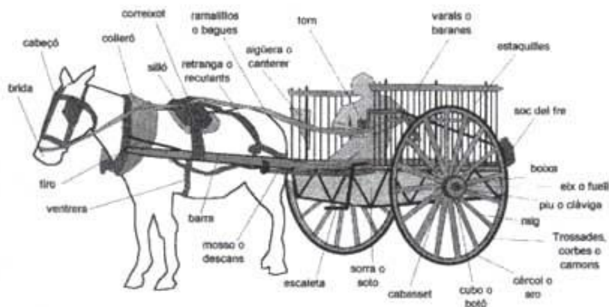
Esquema d'un carro.
