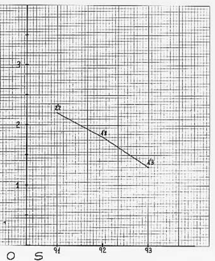
LLUVIAS MEDIAS POR DÍA NATURAL
