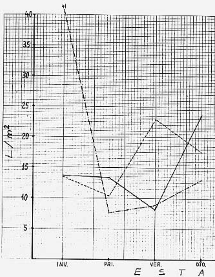
LLUVIAS MEDIAS POR DÍA DE LLUVIA
