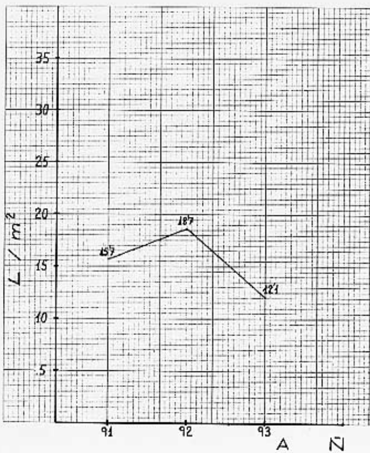
LLUVIAS MEDIAS POR DÍA DE LLUVIA
