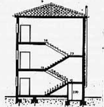
seccion transversal
