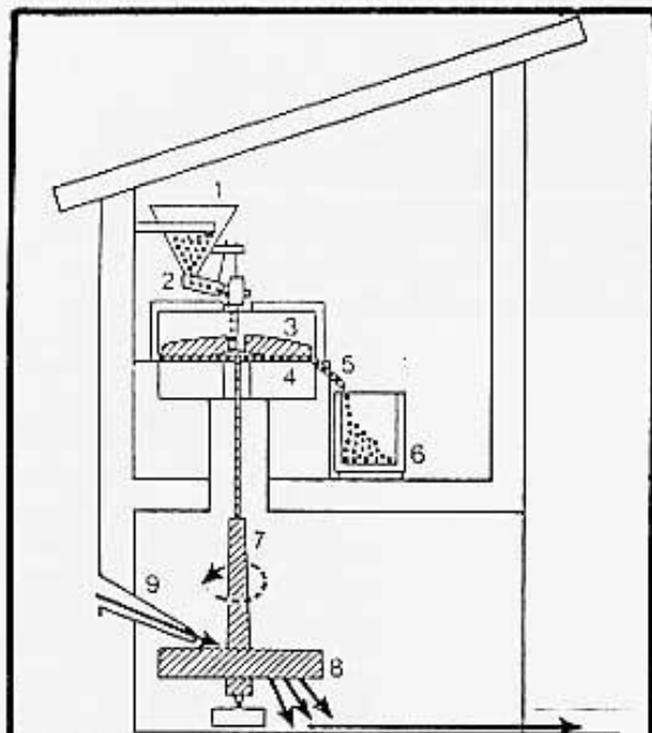
Esquema del funcionament d'un molí fariner. El recorregut del gra i de la farina, representat per punts, comença a la tremuja (1), s'ón passa al canalot (2) que aconduex el gra fins a l'nil de la mola, on cau entremig de la mola volandera (3) i de la mola ratana (4). Un cop el gra és molt surs pel farinal (5) i cau a la farinera (6). El recorregut de l'aigua és representat per sagetes negres. L'aigua de la bassa o del pou surt a pressió per la canal (7) i cau damunt del rodet (8), fent que volti, després s'escala pel sòl del carcau fins a l'exterior. Les peces ratllades: el rodet (8), l'arbre (7) i la mola volandera (3) són les úniques que volten, alhora, en el molí fariner.
